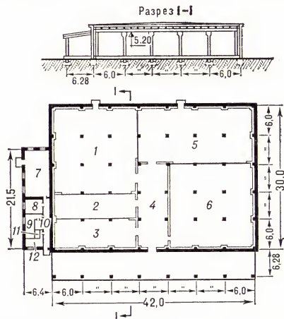
Специализированное плодохранилище ёмкостью 750 т с искусственным охлаждением (размеры в м): 1, 5, 6 — камеры длительного хранения; 2, 3 — камеры предварительного охлаждения; 4 — переборочная; 7 — компрессорная; 8 — электрощитовая; 9, 10, 11, 12 — бытовые помещения.
